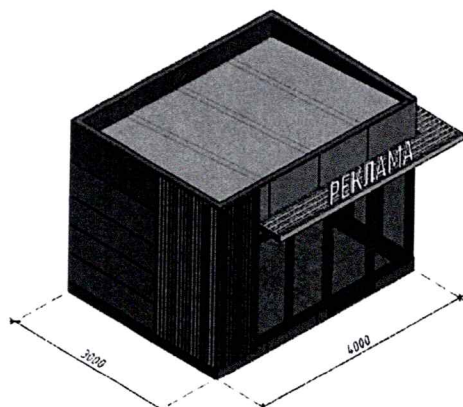
НТО 4х3м
