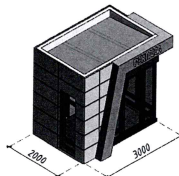
НТО 3x2м
