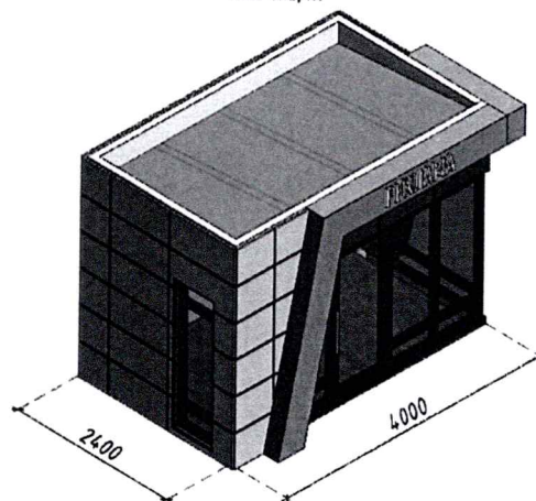
НТО 4x2,4м
