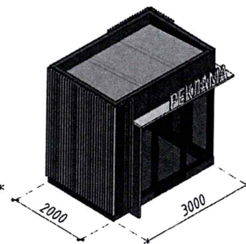
НТО 3x2м
