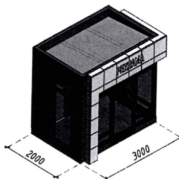
НТО 3x2м
