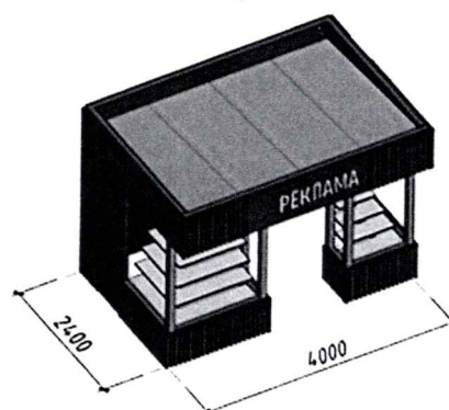
НТО 4х2,4м
